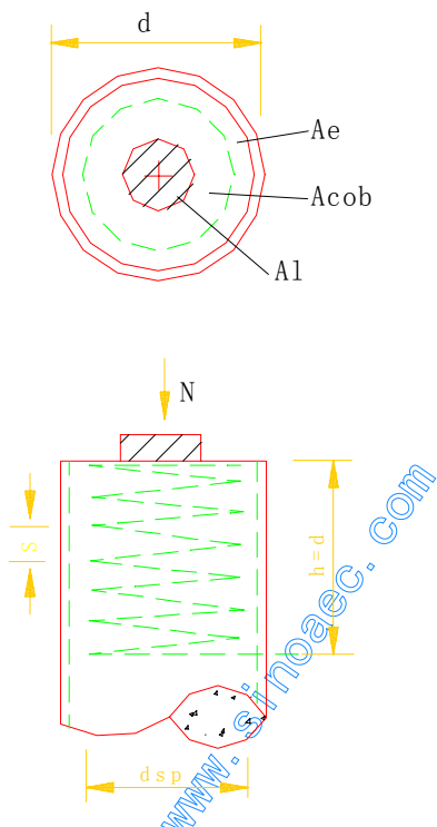
图 4.3.3 配有螺旋箍筋的钢管混凝土局部受压
