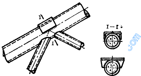
图 6.4.2 上弦节点
