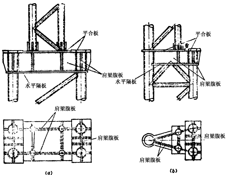
图 6.3.3 阶形格构柱变截面处构造
