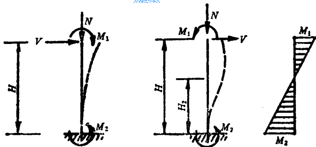
图 4.1.6 悬臂柱
