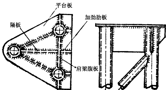
图 6.3.4 边列柱柱端构造
