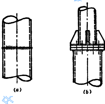
图 6.1.3 钢管接长
