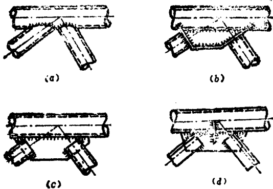
图 6.4.1 杆件节点连接形式
