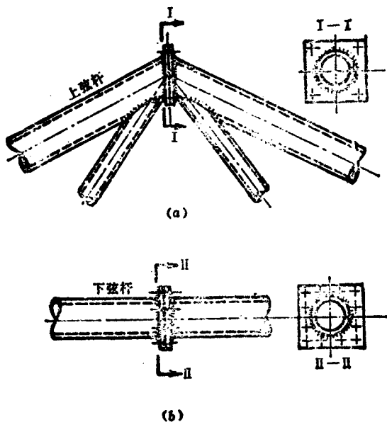
图 6.4.4 跨中安装节点
