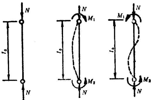
图 4.1.5 无侧移框架柱
