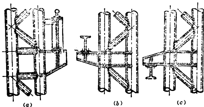
图 6.3.2 等截面格构柱牛腿
