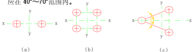
图 4.2.8 格构柱截面
