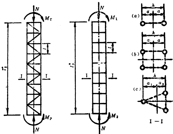
图 4.2.1 格构柱
