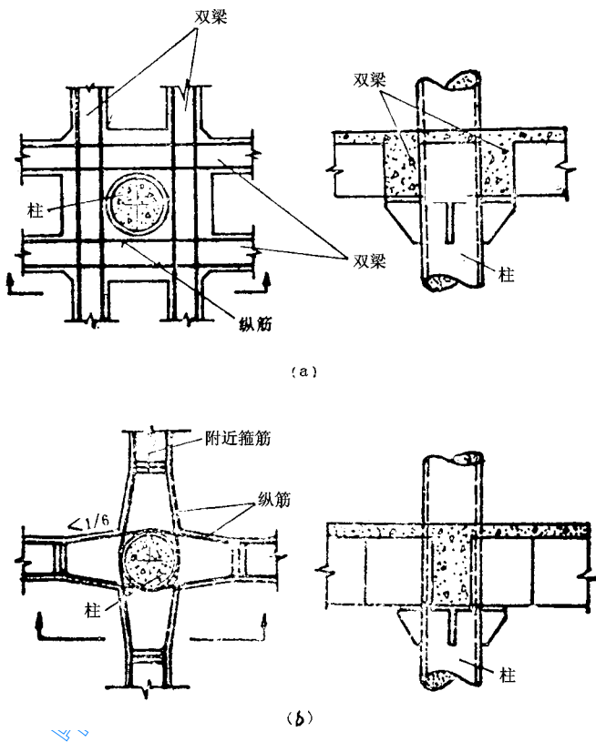
图 6.2.5—2 传递弯矩的梁柱连接
