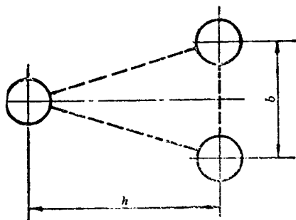
图 6.3.1—1 三肢格构柱截面型式
