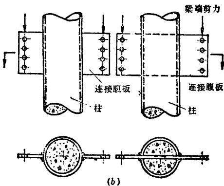
图 6.2.4 传递剪力的梁柱连接 (a) 混凝土梁；(b) 钢梁
