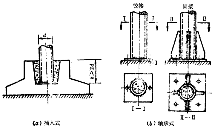
图 6.5.1 柱脚构造
