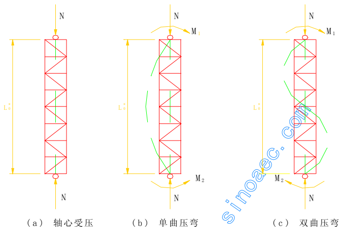
图 4.2.9 格构式无侧移框架柱
