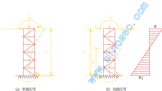
图 4.2.10 格构式悬臂柱
